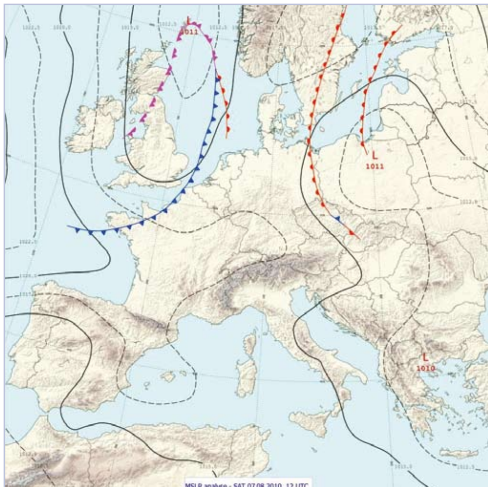
Obr. 5: Analýza tlakového pole a atmosferických front (tlak přepočtený na hladinu moře) dne 7. srpna , 12 UTC
