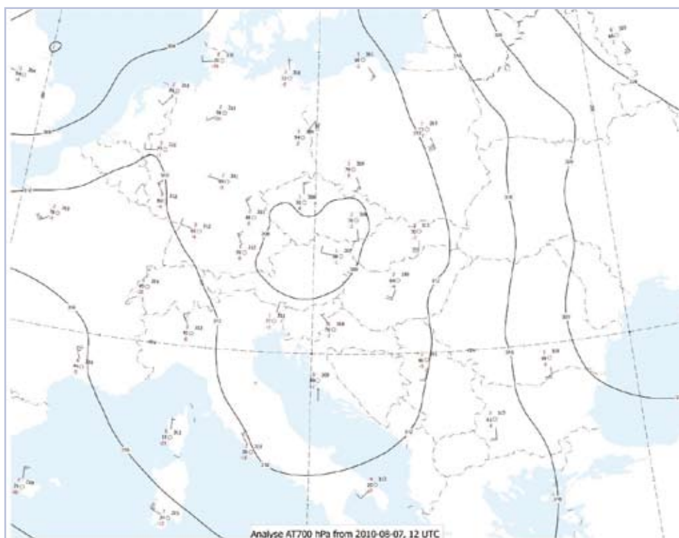
Obr. 6: Analýza tlakového pole v hladině 300 hPa a 700 hPa ze 7. srpna, 12 UTC
